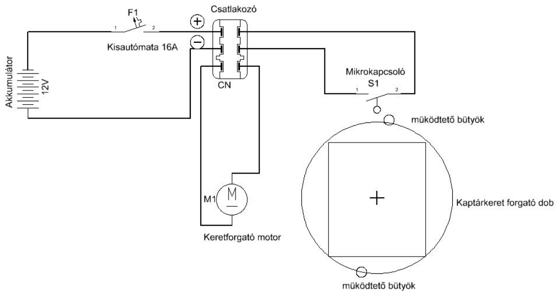
2. ábra A kaptárkeret forgató elektronika bekötése
